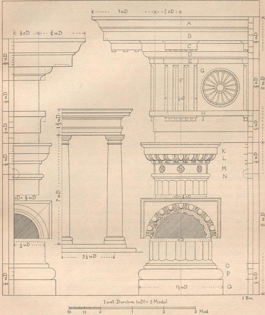
Dorische Ordnung mit Balkenkopfgefmis.
