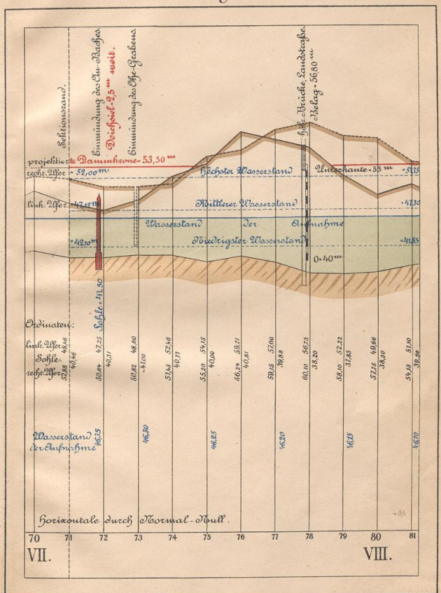
Nivellements - Profile.
