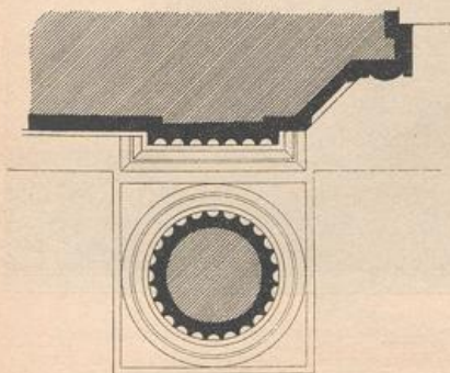
Grundriß zu Fig. 175.
