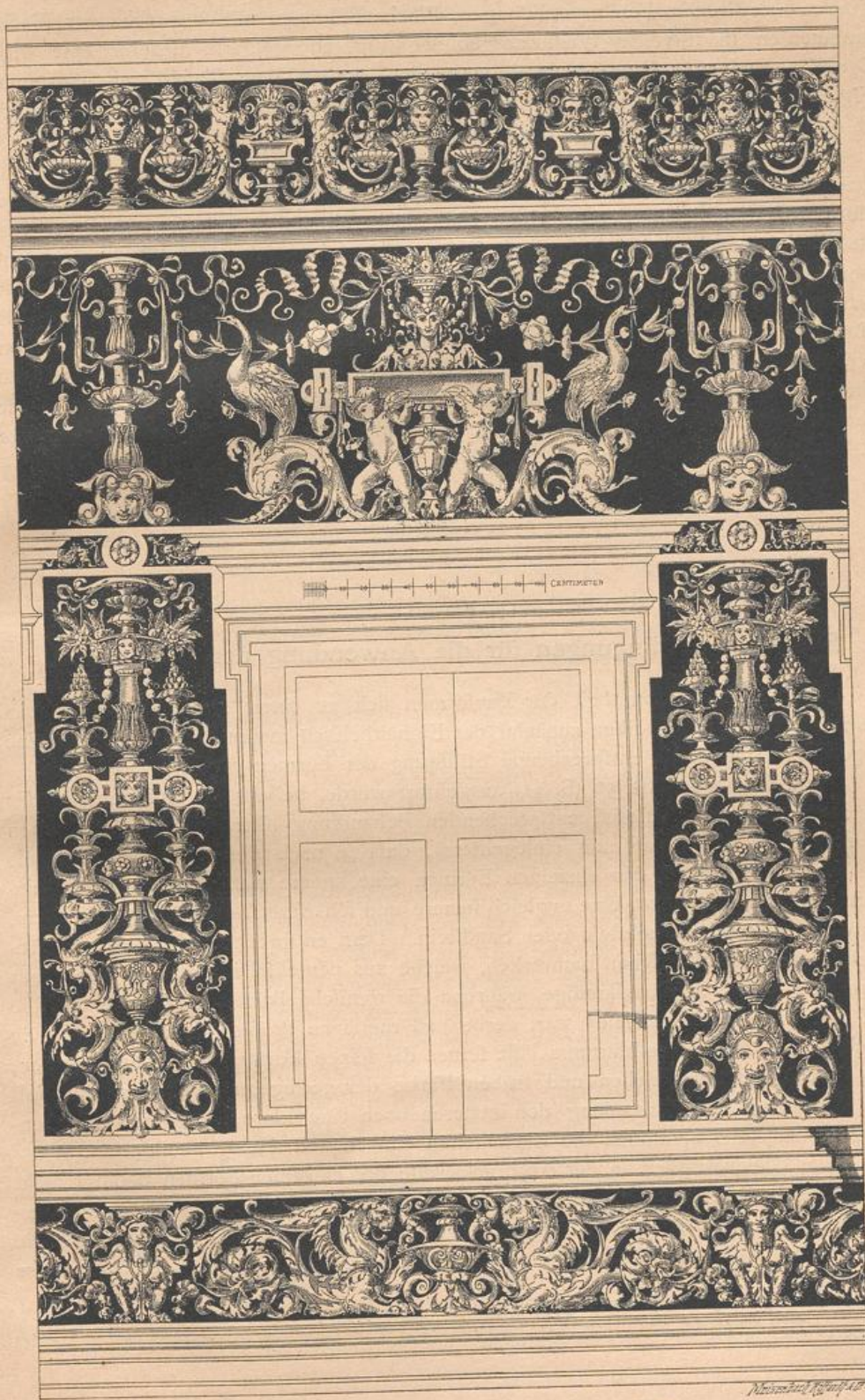
Sgraffito-Decoration vom Palaſt Corsi zu Florenz 142) .
