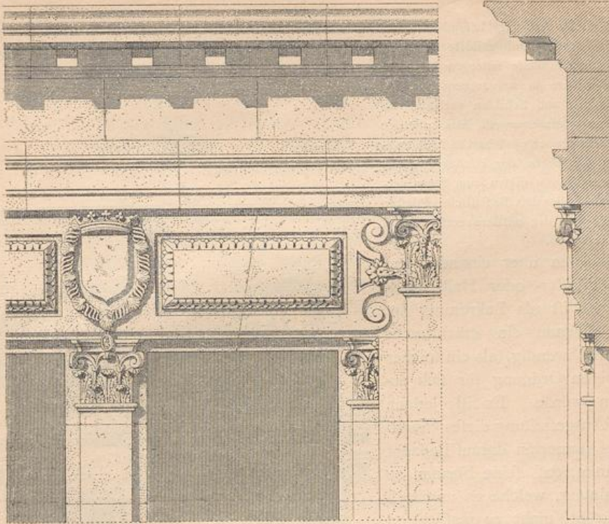
Einzelheiten vom unteren Geschoß in Fig. 227 108 .
