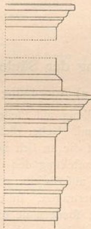
Gebälke und Brüstungsgeims über der unteren Halle 70) .
