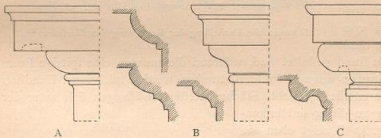
Stützende Wellenleisten.
