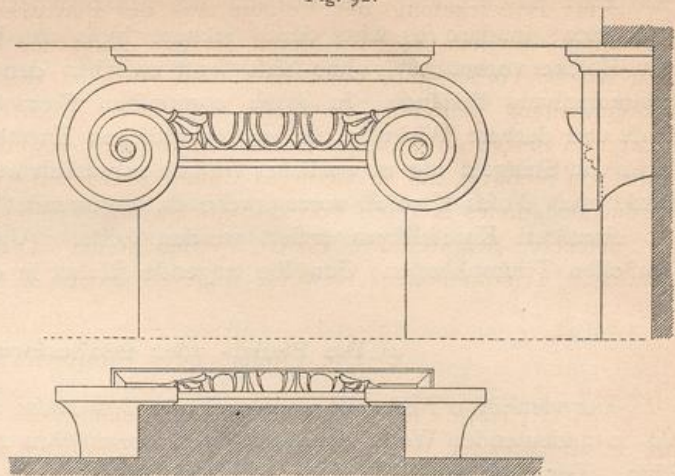
Jonisches Pilaster-Kapitell der Renaissance.
