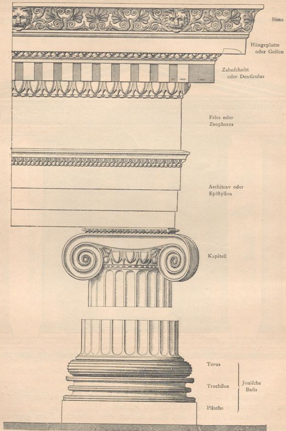
Jonische Ordnung vom Tempel der Athena zu Priene 56) .
