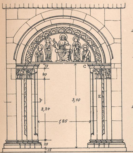
PORTAL IM NÖRDL./SEITENSCHIFF 1:50
