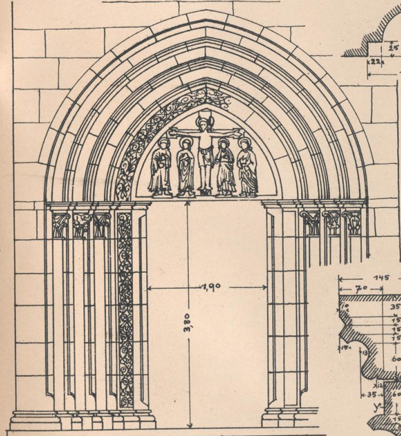
NORDPORTAL IM QERSCHIFF 1:50
