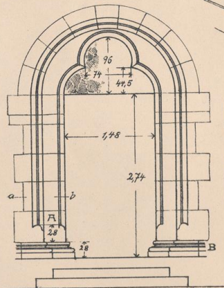
PFARRKIRCHE NEBENPORTAL AN DER SÜDSEITE AUFRISS 1:50 Ä · K
