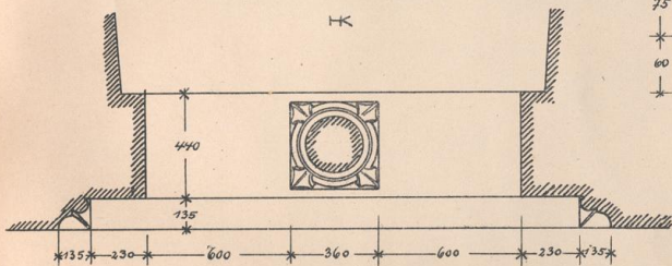
GEKÜPPELTES FENSTER 1:20
