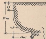
GESIMS 1:10
