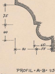
PROFIL A-B 1:5
