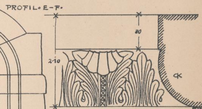
PROFIL E-F
