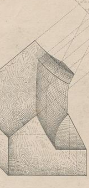
Fig. 259 Isometr. Ansicht des Steines B.
