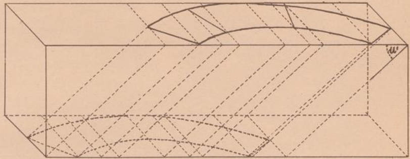
Das Aufreißen der Schablone auf einen Holzblock.
