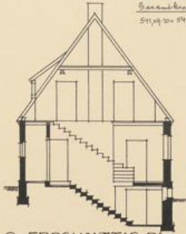
QUERSCHNITT C-D
