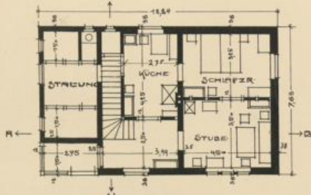
ERDGESCHOSS
