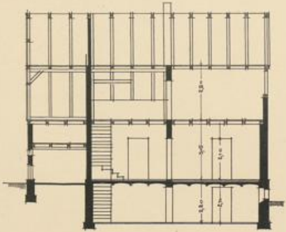
LÄNGSSCHNITT A-B
