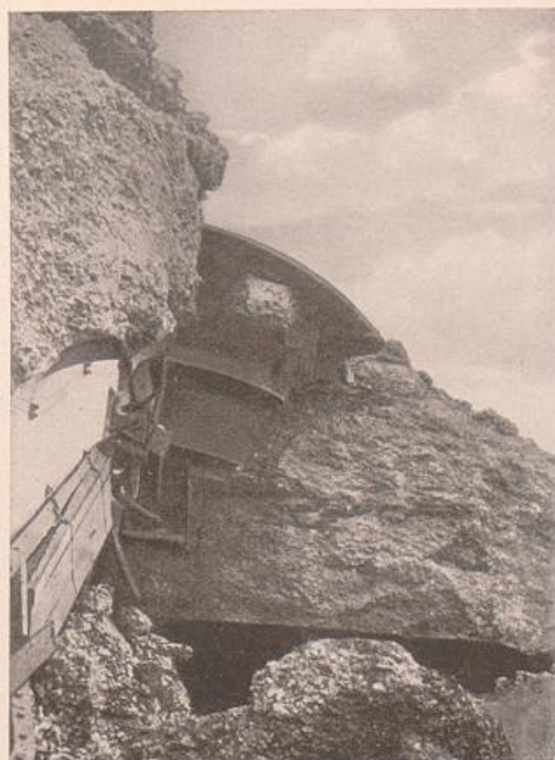
Nr. 59. Wirkung unserer 42 cm-Mörser an den Forts von Lüttich
