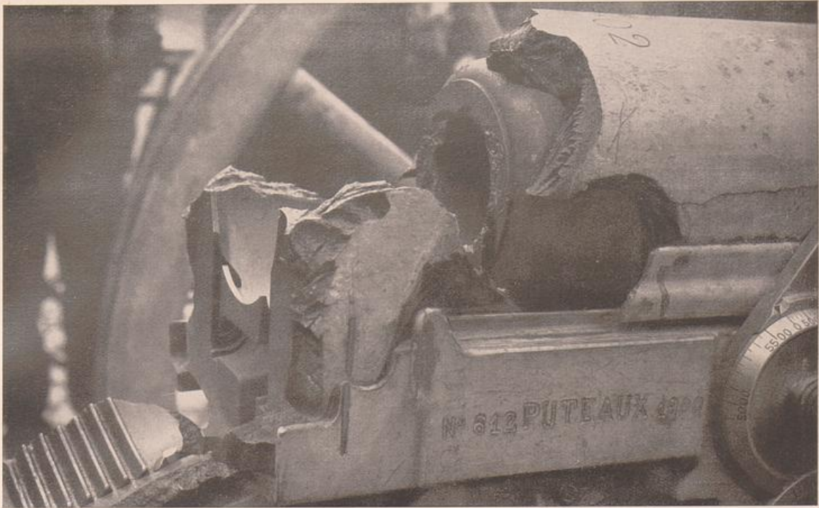
Nr. 117. Furchtbare Explosionswirkung eines deutschen Geschosses am Verschluß und Bronzemantel eines französischen Geschützes
