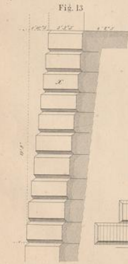
Fig. 11. 13. Umfassungsmauer des Tempels von Jupiter Olympus auf der Ostseite der Akropolis zu Athen.
