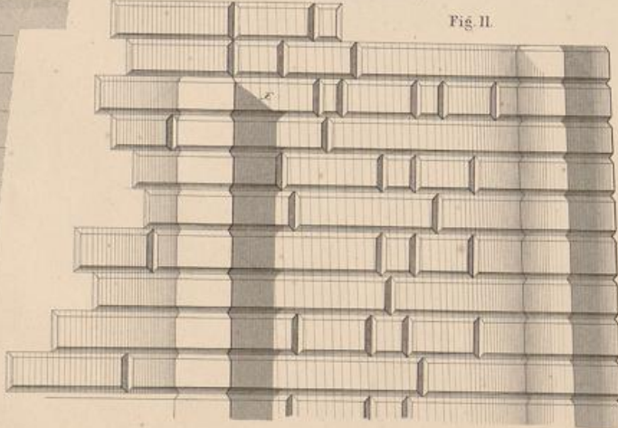
Fig. 11. 13. Umfassungsmauer des Tempels von Jupiter Olympus auf der Ostseite der Akropolis zu Athen.
